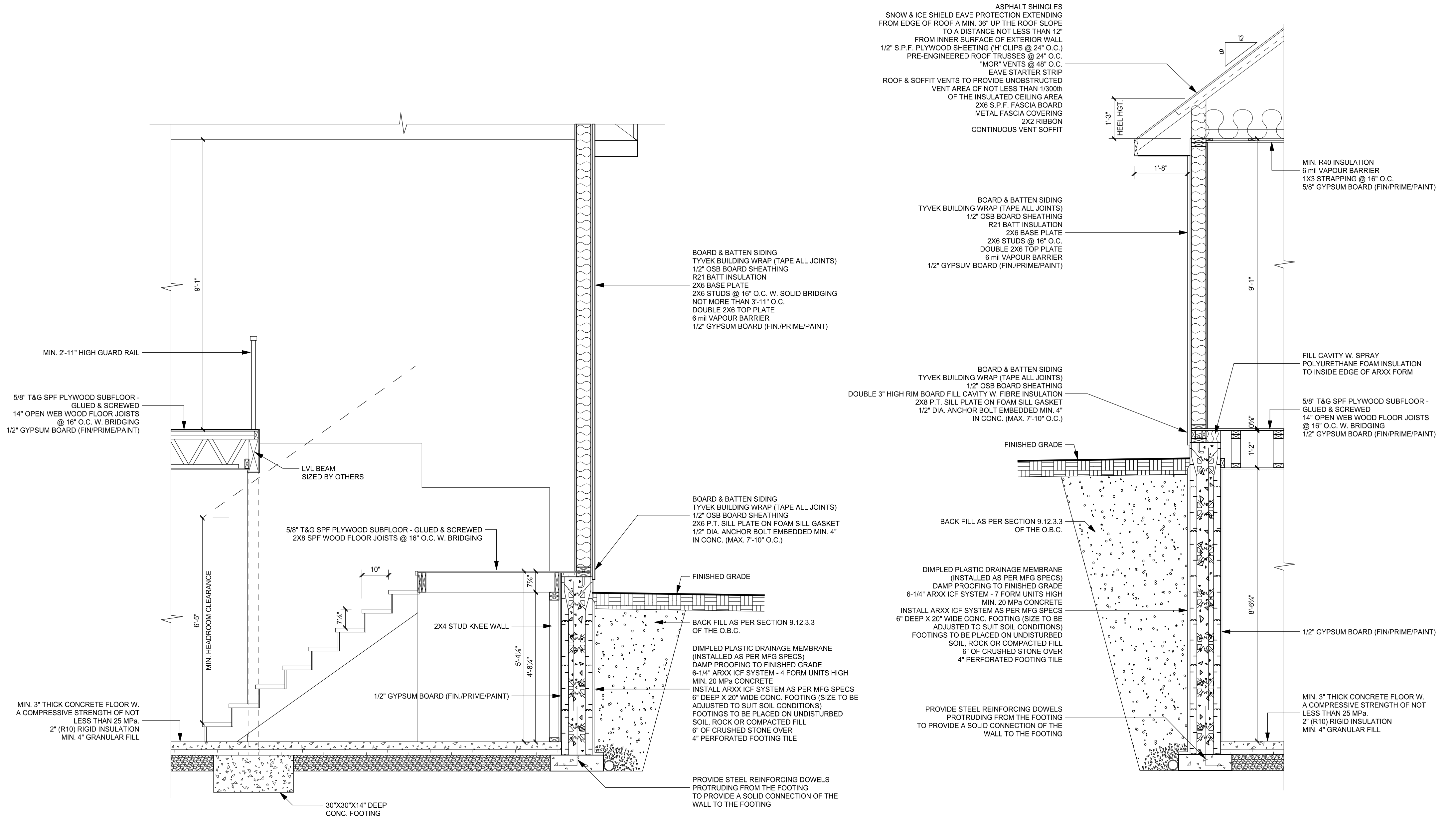
SECTION C SCALE: 1/2" = 1'-0"
